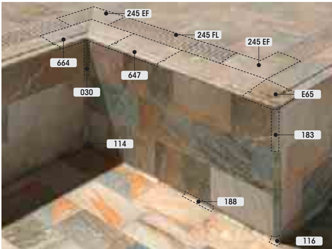
Piscina desbordante / Deck-level pool / Piscine à débordement
