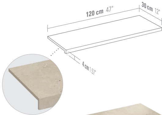
PEÇA DEGRAU LINEAR STEP TREAD
