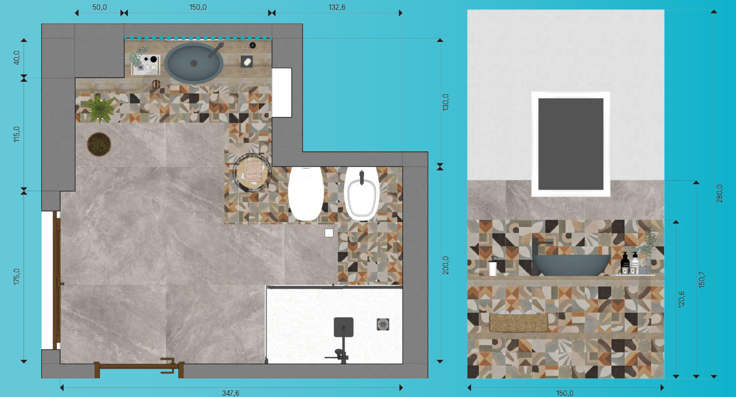
PLANIMETRIA E DETTAGLIO PARETE LAVABO
